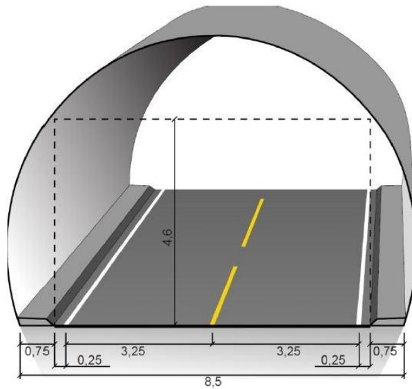
Figur V1.12 Tunnelprofil T8,5 (mål i m)
