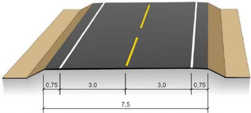
Figur C.5: Tverrrprofil Hø1, 2-feltsveg, vegbreidde 7,5 (mål i m)
