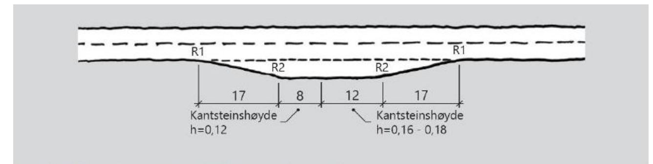
Figur D.38: Busslomme ved utbetningsstandard (mål i m)
